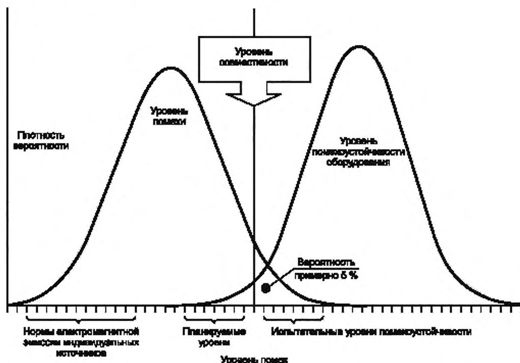
Рисунок А.1 — Уровни электромагнитной эмиссии/помехоустойчивости и уровень совместимости с примером уровней электромагнитной эмиссии/помехоустойчивости для одиночных эмиттера и рецензора как функции некоторых независимых переменных (см. IEC 61000-1-1)
