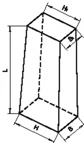
Рисунок 2 – Изделие фасонное номеров 4, 5
