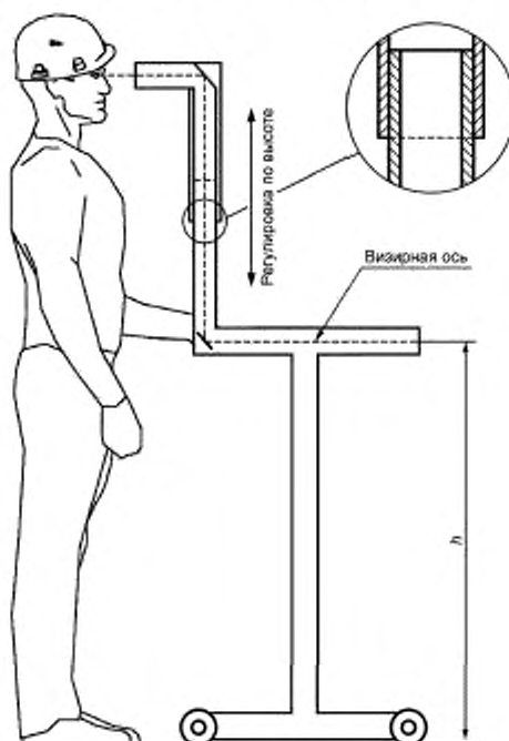
Рисунок А.1 — Схема наблюдения объекта видимости через перископ
