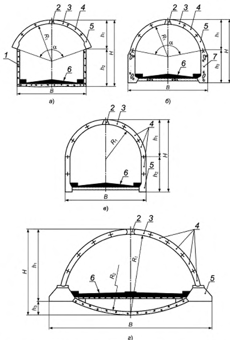
а) в виде полого свода, опирающегося на породу; б) в виде подъемистого свода с бетонными стенами с уширенной пяткой; в) в виде подъемистого свода с плоским лотком; г) в виде арки, опирающейся на бетонные или железобетонные фундаменты; H — высота по оси тоннеля; h_1 — высота свода; h_2 — высота стен; h_3 — высота обратного свода; B — ширина тоннеля; R_1 — радиус свода внутренний; R_2 — радиус обратного свода; \alpha — суммарный угол блоков; 1 — набрызг-бетон; 2 — ключевой блок; 3 — смежный блок; 4 — нормальный блок; 5 — опорный блок; 6 — проезжая часть; 7 — стена из монолитного бетона
