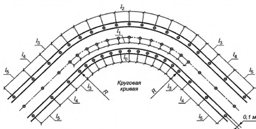
Рисунок 4 — Схема установки световозвращателей типа КДЗ на кривой в плане
