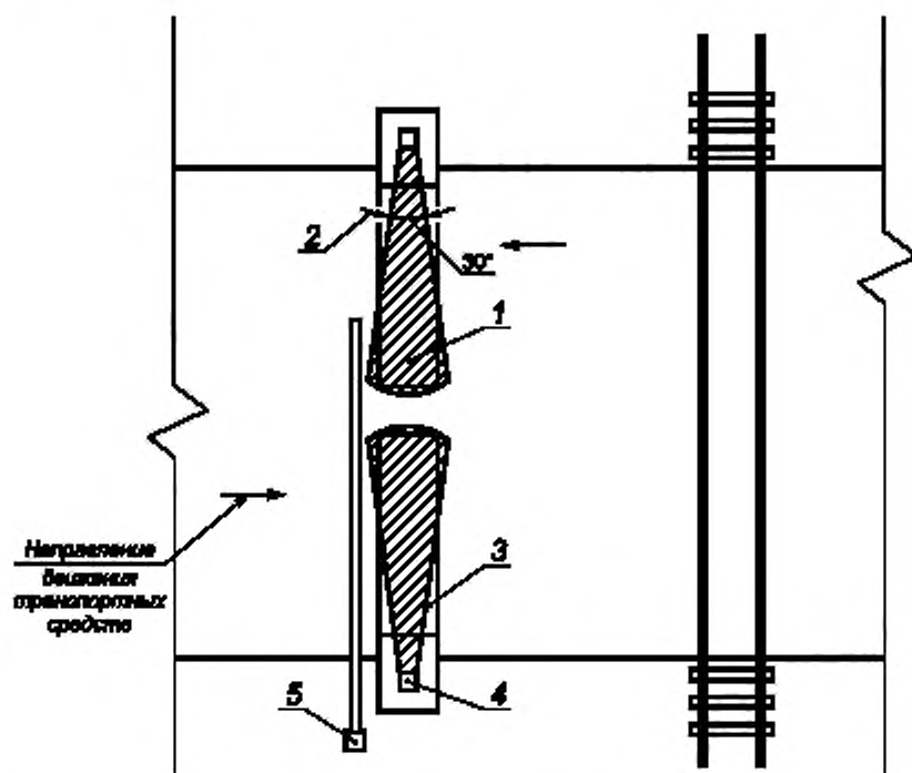
1 — диаграмма направленности; 2 — ширина диаграммы направленности; 3 — крышка ЗД; 4 — КЗК; 5 — шлагдаум
