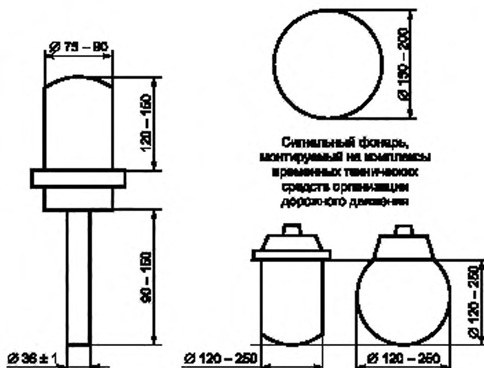
Рисунок 1 — Примеры схем сигнальных фонарей
