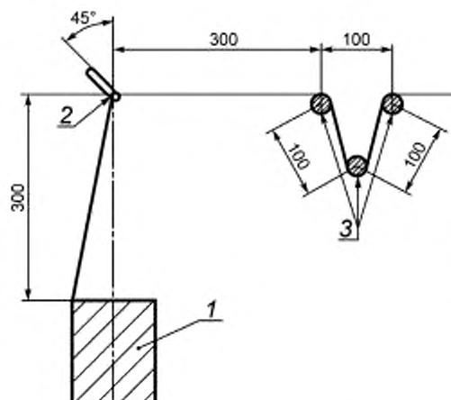
Рисунок 1 — Устройство для контролируемой размотки ровинга
