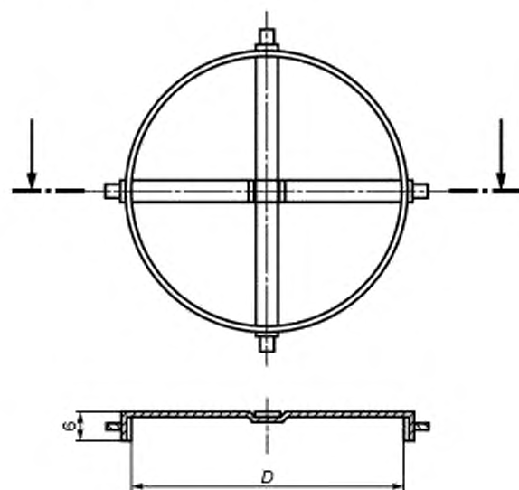
a – Кольцевой трафарет
