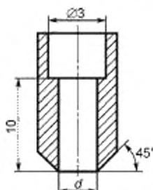
Исполнение I, применяемое для внутренних диаметров насадки не более 3 мм
