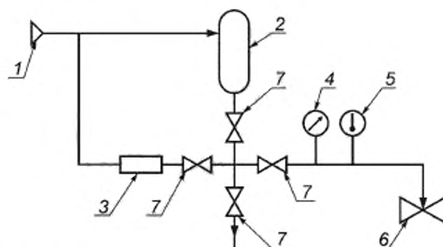
1 — источник испытательной среды; 2 — источник давления; 3 — напорно-расходомерное устройство; 4 — прибор для измерения давления; 5 — термометр; 6 — испытуемая арматура; 7 — запорно-регулирующий клапан
