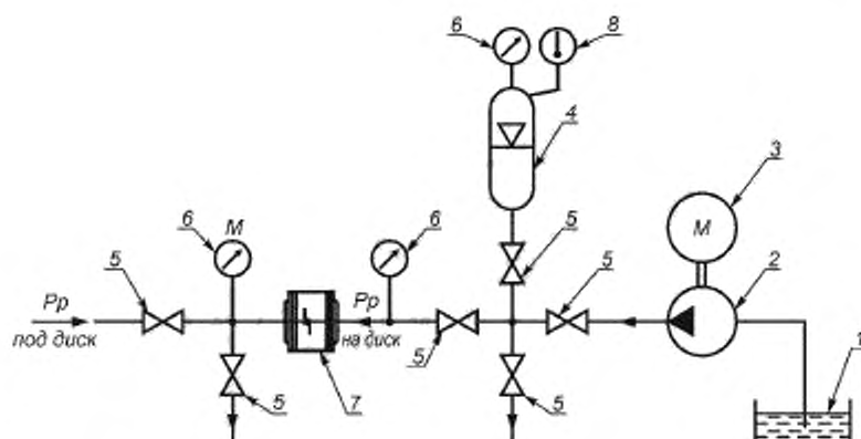
1 — бак; 2 — насос (допускается применять другие технические средства); 3 — электродвигатель; 4 — гидропневмоаккумулятор; 5 — запорно-регулирующий клапан; 6 — прибор для измерения давления; 7 — испытуемая арматура; 8 — термометр
