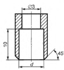
Исполнение II, применяемое для внутренних диаметров насадки более 3 мм
