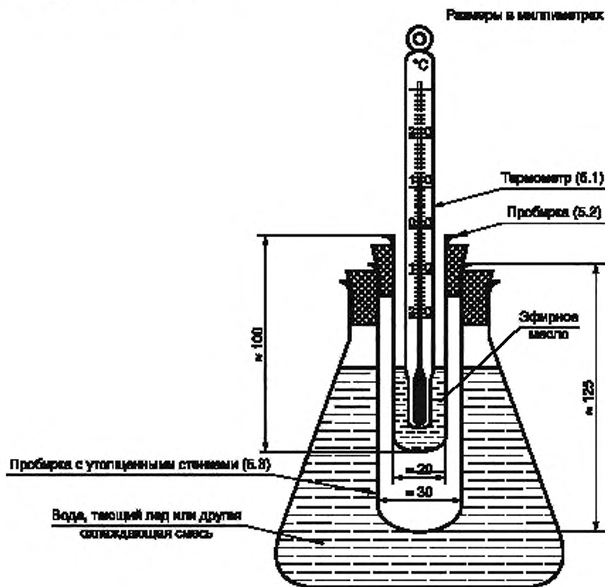
Рисунок — Подходящий прибор для определения температуры застывания
