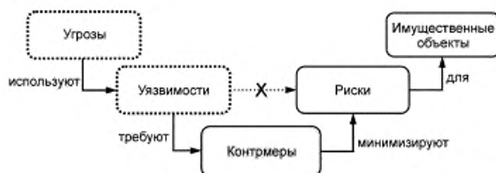
Рисунок 1 — Взаимосвязь угроз-рисков
