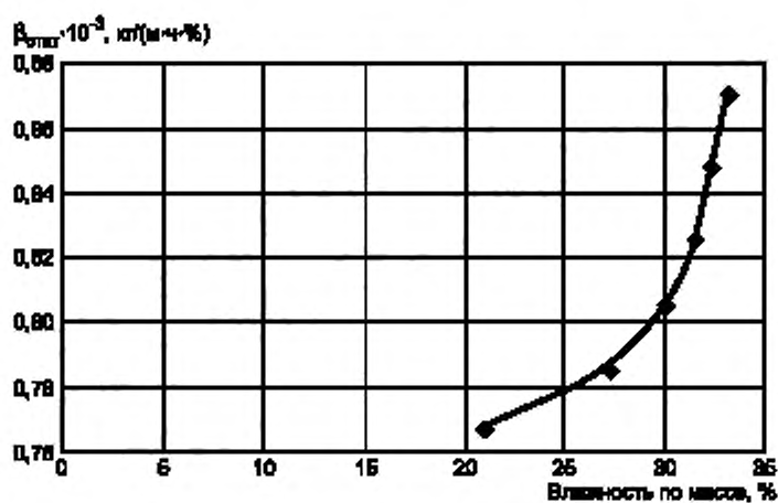
Рисунок А.3 — Зависимость коэффициента статической влагонепроводности газобетона марки по средней плотности D500 от влажности
