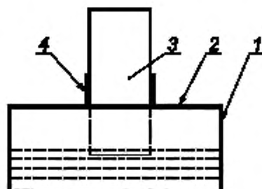
1 — контейнер с водой; 2 — крышка контейнера; 3 — образец; 4 — герметик
