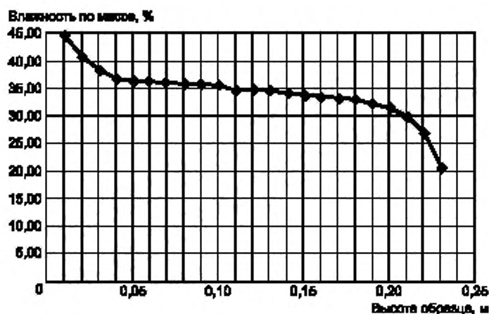
Рисунок А.1 — Распределение влажности по высоте образца
