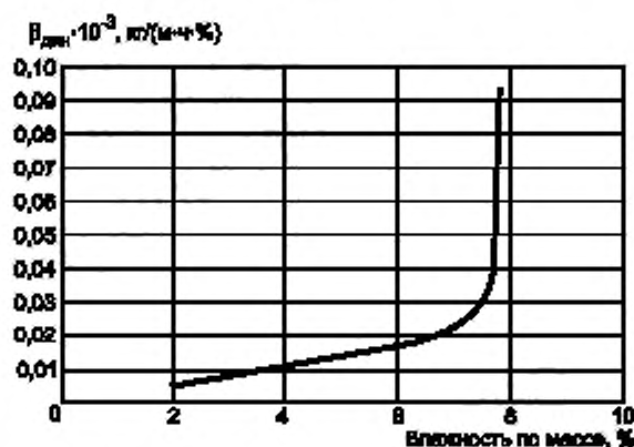
Рисунок Б.1 — Зависимость коэффициента динамической влапопроводности штукатурного состава от влажности
