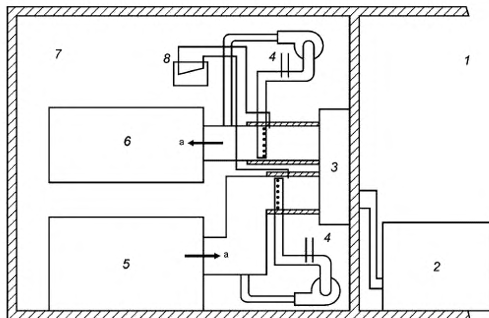
1 — отсека наружной стороны; 2 — наружный блок испытываемого оборудования; 3 — внутренний блок испытываемого оборудования; 4 — измерительные приборы температуры и влажности; 5 — аппарат повторного кондиционирования; 6 — аппаратура измерения воздушного потока; 7 — отсека внутренней стороны; 8 — аппаратура измерения перепада давления; а — воздушный поток
