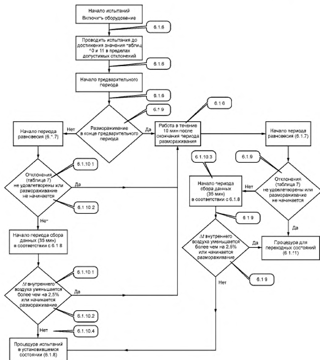
Рисунок H.1 — Блок-схема процедуры
