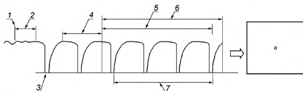
1 — достигнуто соответствие с допустимыми отклонениями испытания; 2 — период предварительной подготовки (минимально — 10 мин); 3 — размораживание в конце периода предварительной подготовки; 4 — период равновесия (60 мин); 5 — период сбора данных; 6 — 3 ч; 7 — три полных цикла размораживания; а — завершить испытание, когда период сбора данных равен 3 ч
