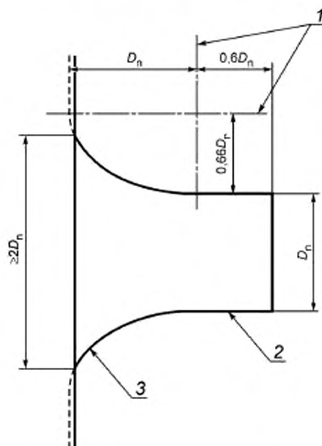
1 — ось эллипса; 2 — секция горловины; 3 — эллиптическая кривая; D_n — диаметр горловины сопла, м
