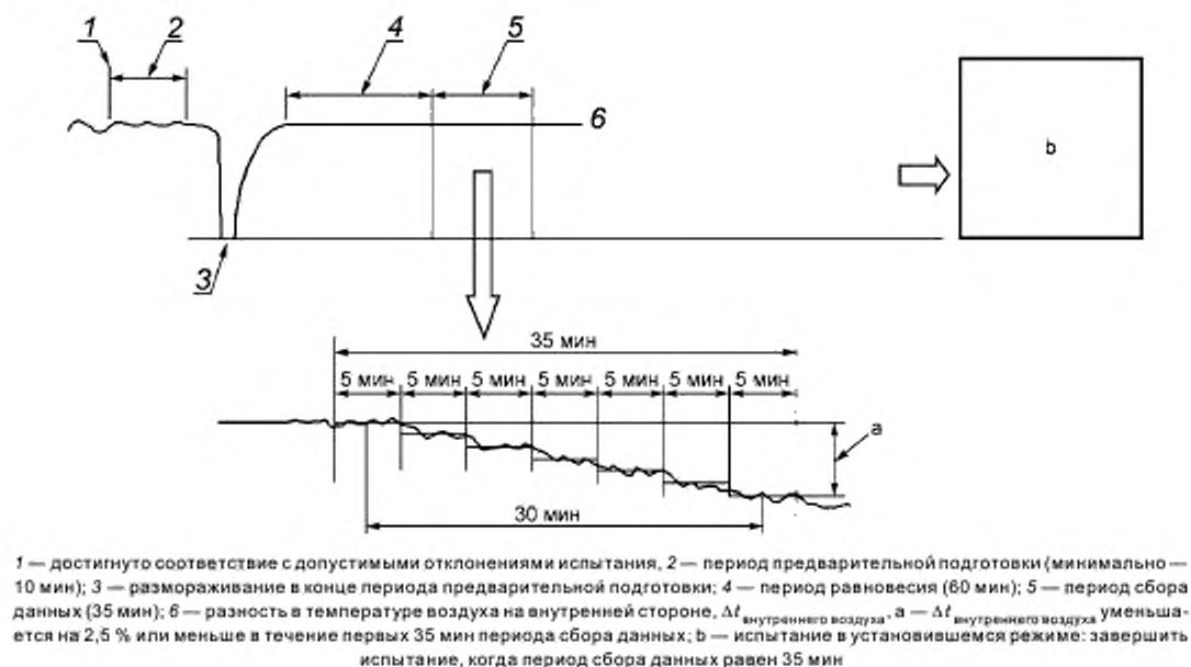
Рисунок Н.2 — Испытание теплопроводности в установившемся режиме
