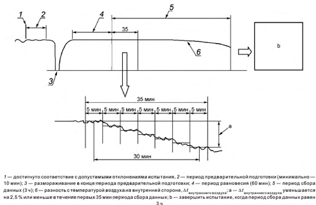
Рисунок Н.3 — Испытание теплопроводности в режиме переходного процесса без циклов размораживания
