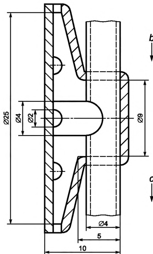
Рисунок 4 — Пробоотборник
