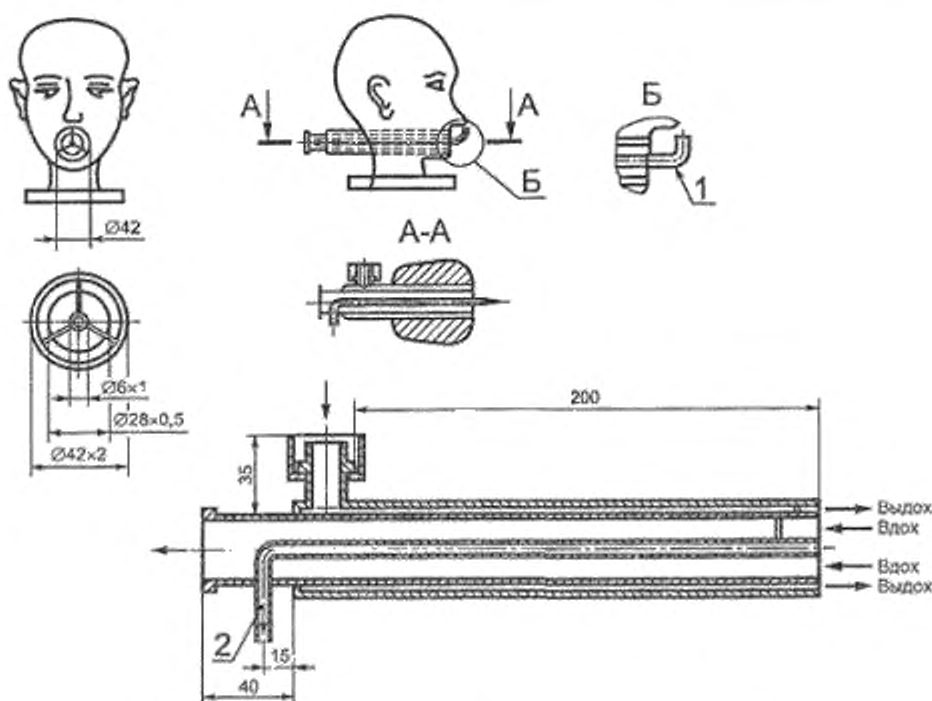
1 — адаптер для измерения сопротивления воздушному потоку; 2 — измерение \text{CO}_2 на (вдохе)
