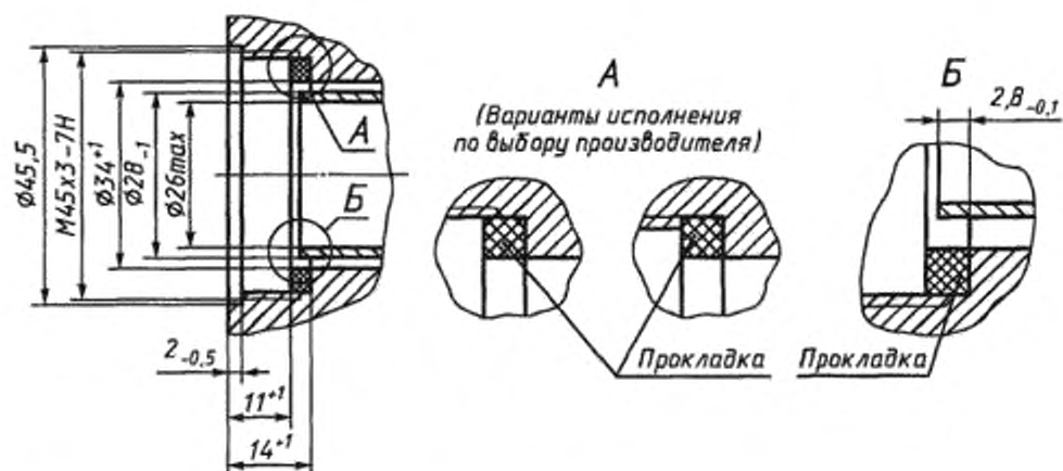
Рисунок Б.4 — Резбовое соединение с внутренней резьбой для систем с двумя каналами подачи воздуха PIB
