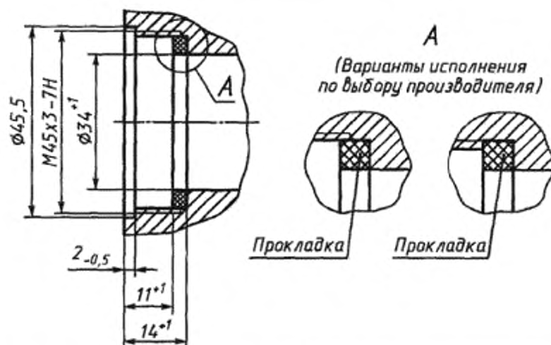
Рисунок Б.3 — Резьбовое соединение с внутренней резьбой для систем с одним каналом подачи воздуха PIA
