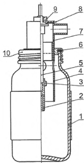
Рисунок 12 — Установка для определения коэффициента подсоса под маску
