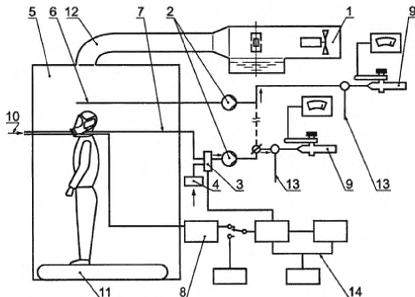
1 — генератор аэрозоля; 2 — сопло; 3 — клапан переключения; 4 — фильтр; 5 — испытательная камера; 6 — отбор пробы из испытательной камеры; 7 — отбор пробы из подмасочного пространства маски; 8 — манометр; 9 — фотометр; 10 — имитатор фильтрационного воздуха; 11 — тредбан; 12 — трубопровод и распределитель потока; 13 — дополнительная подача воздуха; 14 — система разделения фаз вдоха-выдоха при отборе проб
