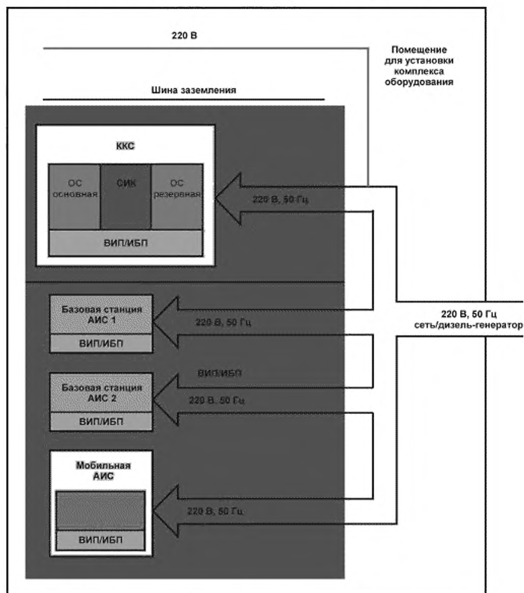
Рисунок 2 — Схема электропитания комплекса оборудования «ККС — БС — АИС» и «АИС транспондера»
