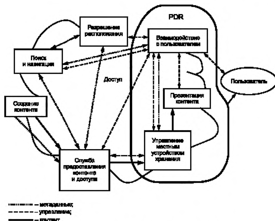
Рисунок 2 — Полная интерактивная модель системы TV-Anytime
