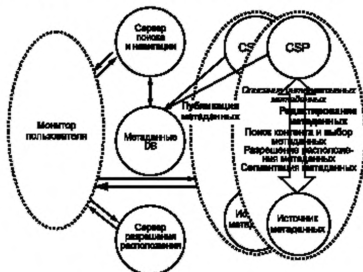
Рисунок 14 — Двунаправленная транспортировка метаданных
