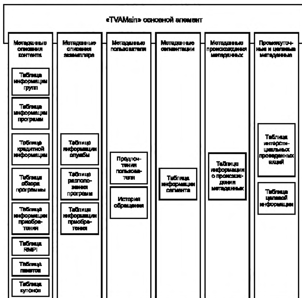
Рисунок 6 — Документы TV-Anytime с корневым элементом «TVAMail»
