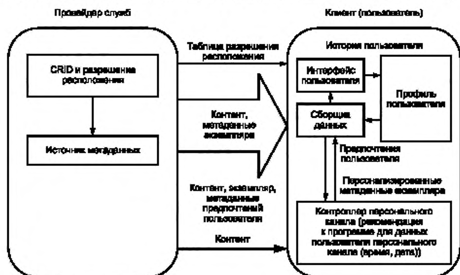
Рисунок 12 — Операции взаимодействия между провайдером служб и пользователем
