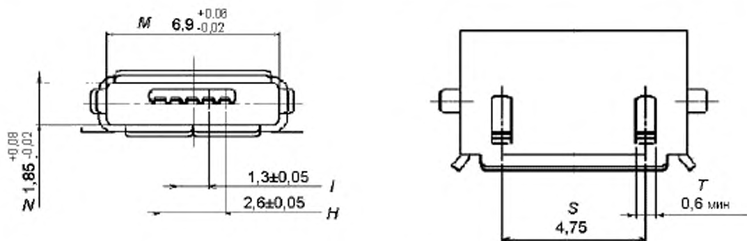
Рисунок В.8.1 — Габаритные размеры USB серии «Микро «AB» — розетка
