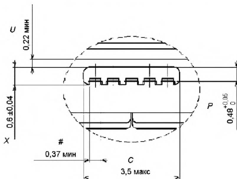
Рисунок В.8.2 — Габаритные размеры USB серии «Микро «AB» — розетка
