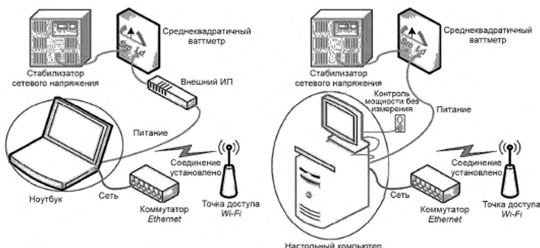
Рисунок 1 — Типичная испытательная установка
