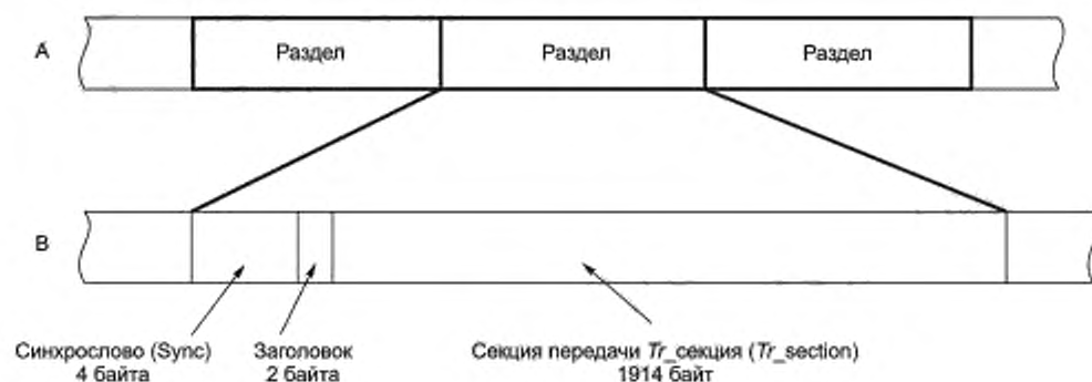
Рисунок 14 — Поток передачи
