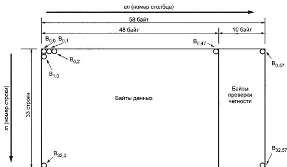
Рисунок 7 — Структура блока
