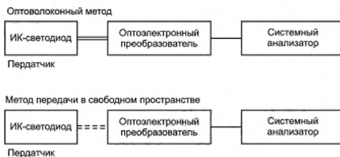
Рисунок 32 — Система измерения паразитного излучения
