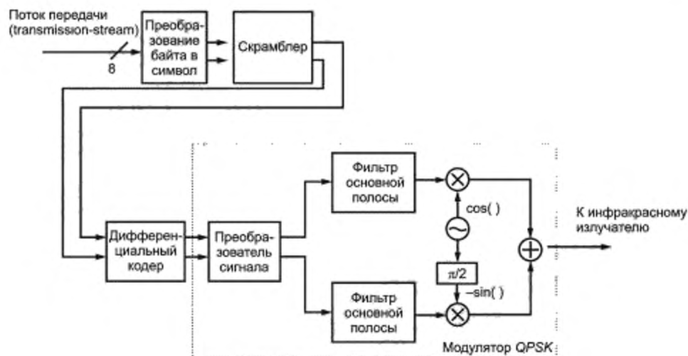
Рисунок 16 — Блок модуляции
