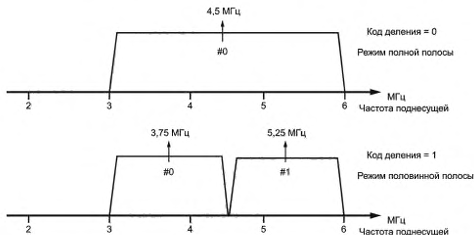
Рисунок 6 — Распределение каналов
