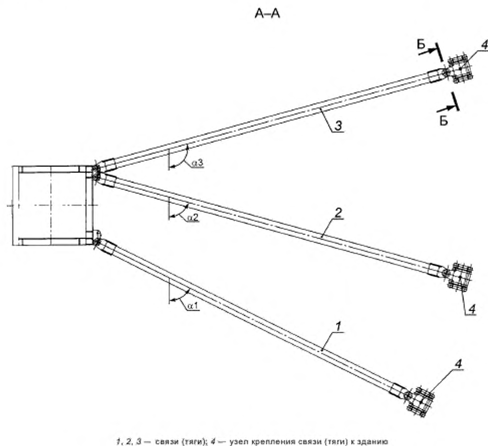
Рисунок 2 — Пример схемы расположения связей горизонтальной опоры в плане
