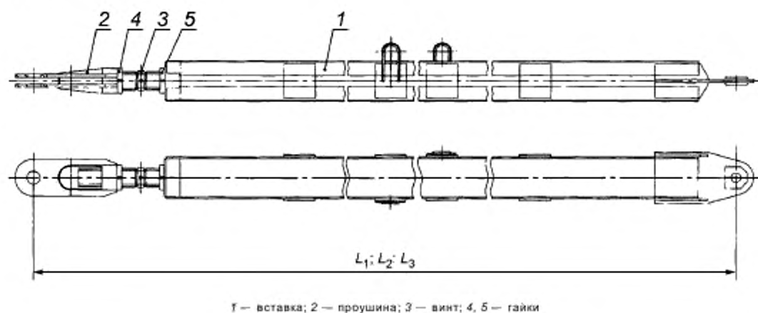
Рисунок 4 — Пример конструкции связи (тяги) (без узлов крепления)
