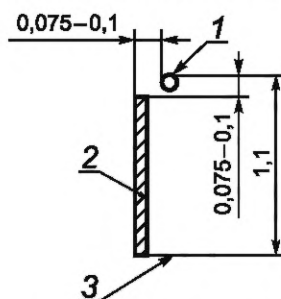
1 — поручень; 2 — боковое ограждение; 3 — пол (настил) кабины (люльки)
