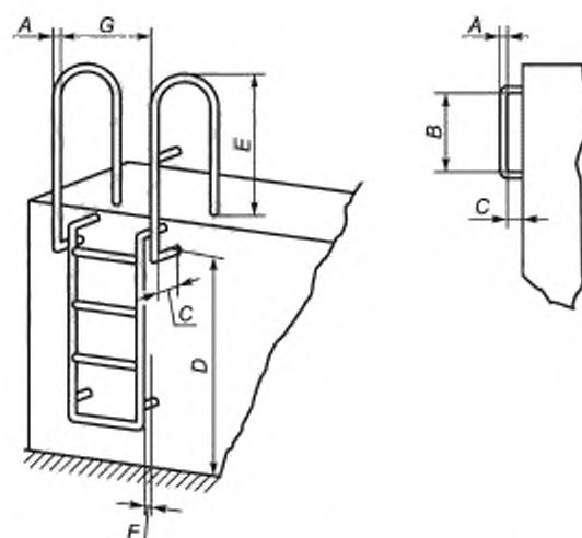
Рисунок А.1 — Перила и поручни
