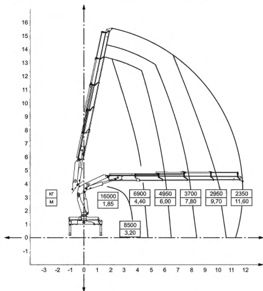
Рисунок 3 — Пример грузовой характеристики
