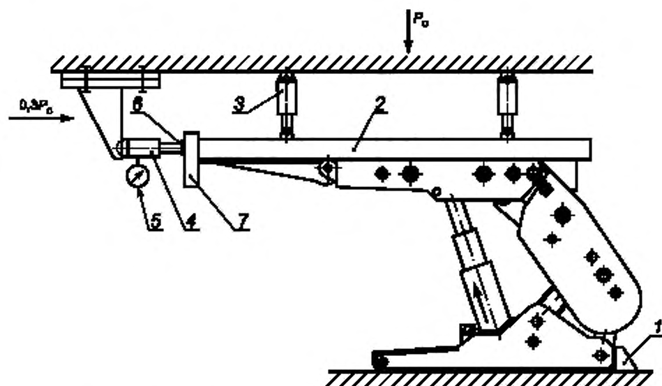
1 — упор; 2 — рама; 3, 4 — гидродомкраты; 5 — манометр; 6 — тензодатчик; 7 — упор
