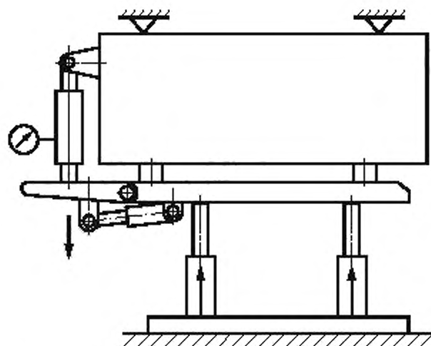
Рисунок В.3 — Схема нагружения для определения сопротивления на конце гидродожимной консоли (козырька) перекрытия
