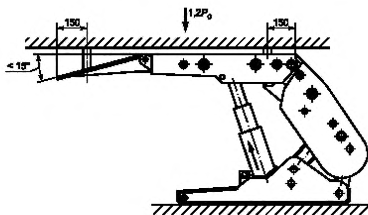
Рисунок Г.1 — Схема испытания перекрытия с поджимной консолью, замыкающейся «на жестко»
