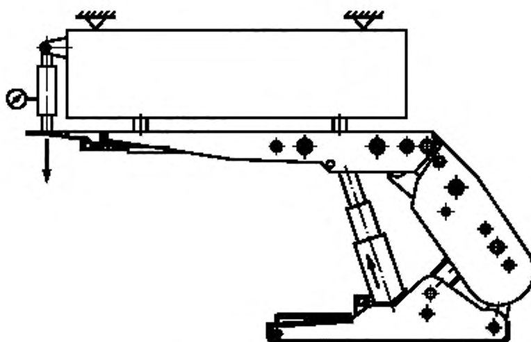
Рисунок В.4 — Схема нагружения для определения сопротивления на конце составной гидродожимной консоли перекрытия
