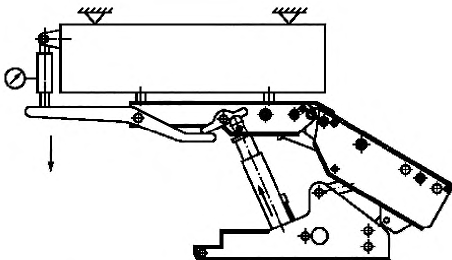
Рисунок В.6 — Схема нагружения для определения сопротивления на конце гидродожимной консоли перекрытия рычажного типа
