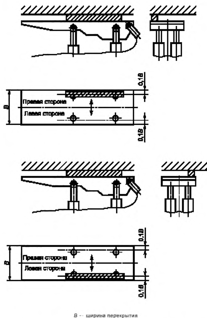
Рисунок Л.1 — Схемы испытаний на внецентренную нагрузку четырёхстоечной секции крепи
