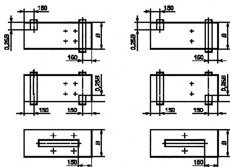
Рисунок Е.1 — Схемы нагружения жесткой балки перекрытия при испытании на изгиб с кручением
