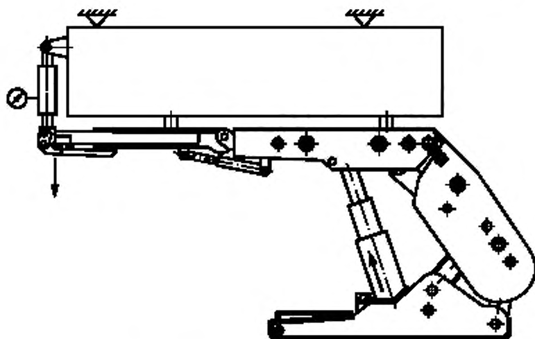
Рисунок В.5 — Схема нагружения для определения сопротивления на конце гидродожимной консоли перекрытия пенального типа
