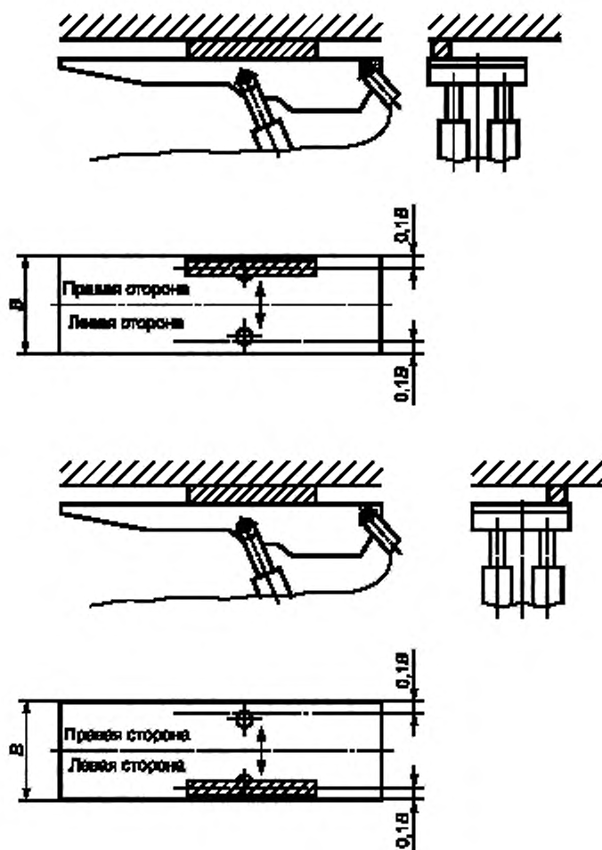
Рисунок Л.2 — Схемы испытаний на внецентренную нагрузку двухрядной секции крепи
