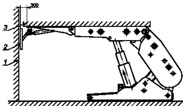
Рисунок И.1 — Схема нагружения механизма удержания забоя
