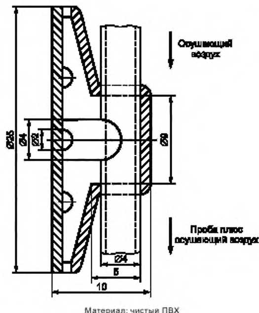
Рисунок 5 — Пробоотборник
