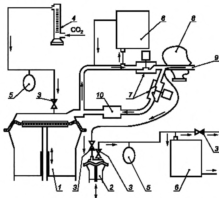
1 — дыхательная машина; 2 — вспомогательное «клеточное»; 3 — обратный клапан; 4 — расходомер; 5 — компенсатор; 6 — анализатор диоксида углерода; 7 — соленоидные клапаны; 8 — голова манекена; 9 — трубка для отбора проб из вдыхаемого воздуха; 10 — поглотитель диоксида углерода
