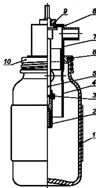
1 — стеклянный сосуд с навинчивающейся крышкой; 2 — солло; 3 — волокнистая прокладка (наружный диаметр — 4,5 мм, внутренний диаметр — 2 мм, толщина прокладки — 0,8 мм); 4 — втулка; 5 — стержень; 6 — резиновая прокладка; 7 — головка втулки; 8 — резиновая прокладка (наружный диаметр — 25 мм, внутренний диаметр — 10 мм, толщина — 1,5 мм, уплотнитель для герметизации); 9 — гайка; 10 — навинчивающаяся крышка
