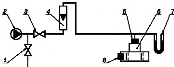
1, 3 — регулирующие вентили; 2 — устройство подачи воздуха; 4 — расходомер с верхним пределом измерения 0,063 м³/ч и приведенной погрешностью не более ± 2,5 %; 5 — присоединительное устройство; 6 — клапанная коробка; 7 — мановакуумметр с пределом измерения до 2500 Па и абсолютной погрешностью не более ± 20 Па, 8 — пробка
