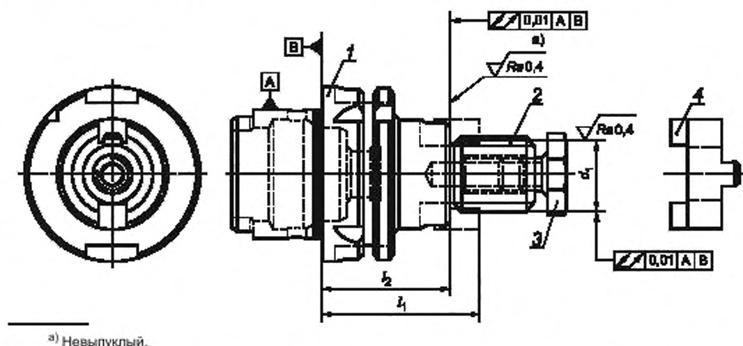
1 — полый конический хвостовик HSK; 2 — шпоночный паз, шпонка; 3 — зажимной винт для фиксации фрезы; 4 — поводок
