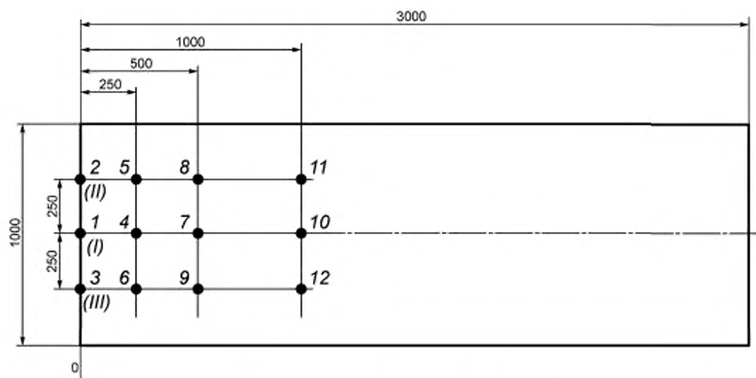
Рисунок А.2 — Схема размещения термодатчиков на поверхности калибровочного образца, а также на поверхности образца покрытия и места измерения скорости направленного потока воздуха
