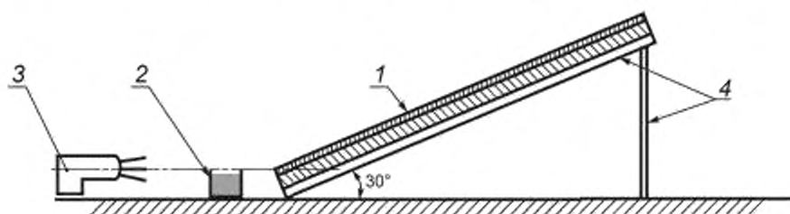
Рисунок А.2 — Схема размещения термодатчиков на поверхности калибровочного образца, а также на поверхности образца покрытия и места измерения скорости направленного потока воздуха
