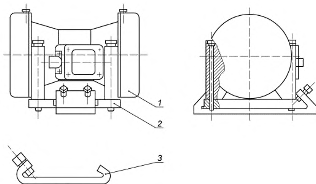
а) Направляющая типа «ласточкин хвост»
