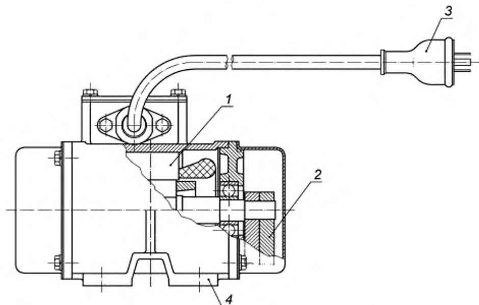
1 — статор электродвигателя; 2 — дебаланс; 3 — штепсельная вилка; 4 — станина
