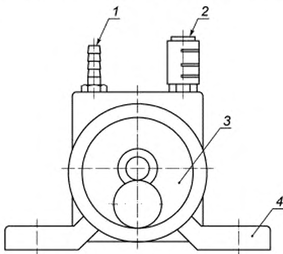
1 — шланг; 2 — глушитель; 3 — шарнир; 4 — станина
