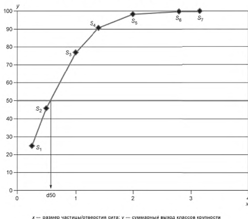
Рисунок А.1 — Графическое отображение среднего размера частиц пробы древесных опилок (результаты ситового анализа приведены ниже)
