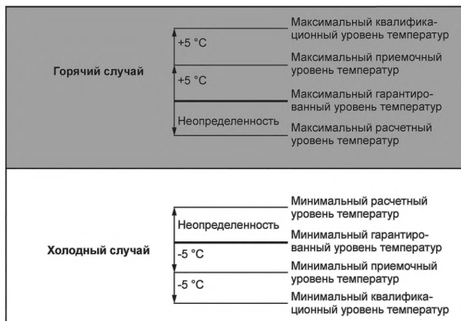
Рисунок 1 — Схема распределения диапазонов квалификационных, приемочных и расчетных температур
