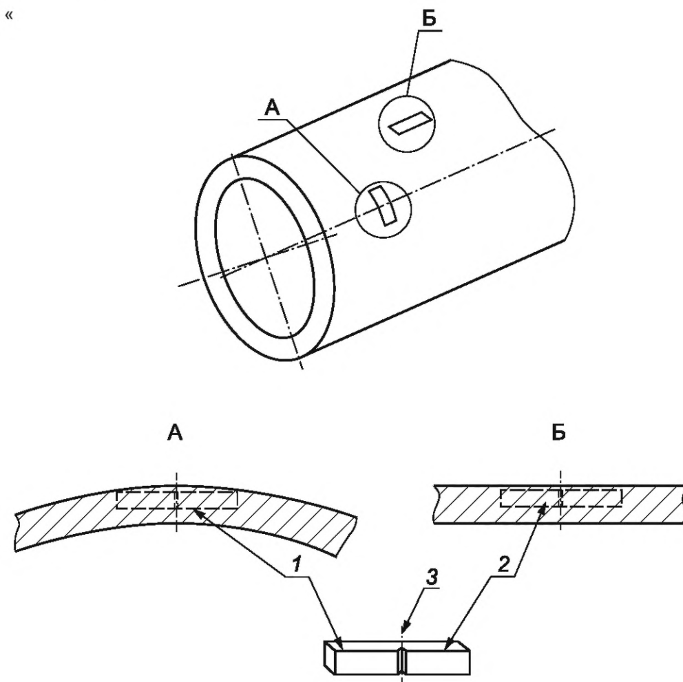
1 — проба для изготовления поперечного образца для испытания; 2 — проба для изготовления продольного образца для испытания; 3 — ось надреза
