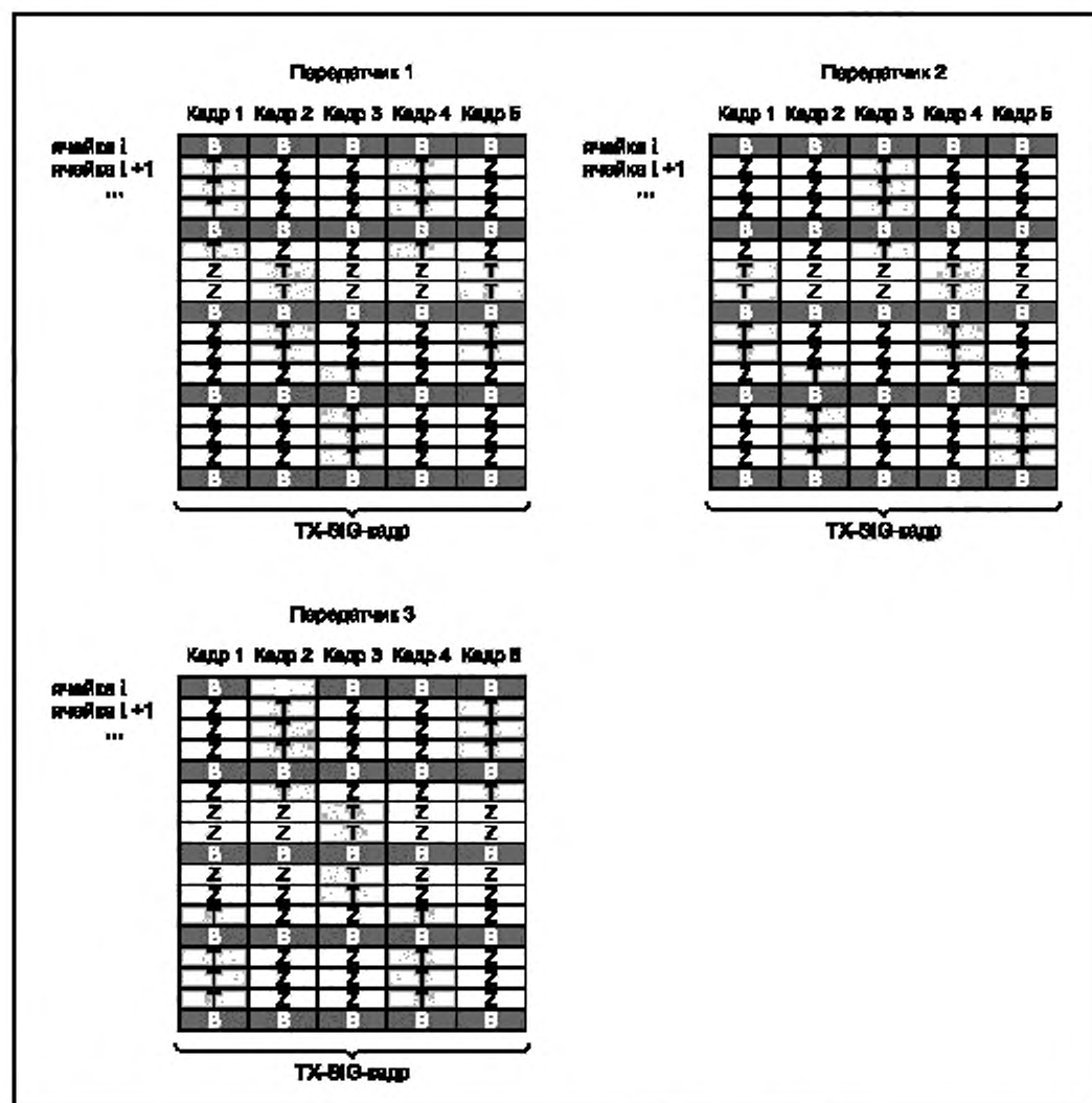
Рисунок 2 — Пример шаблонов дополнительных ячеек, содержащих сигнатуры передатчиков, после вставки В-ячеек, для случая M = 3 , N = 4 , L = 5
