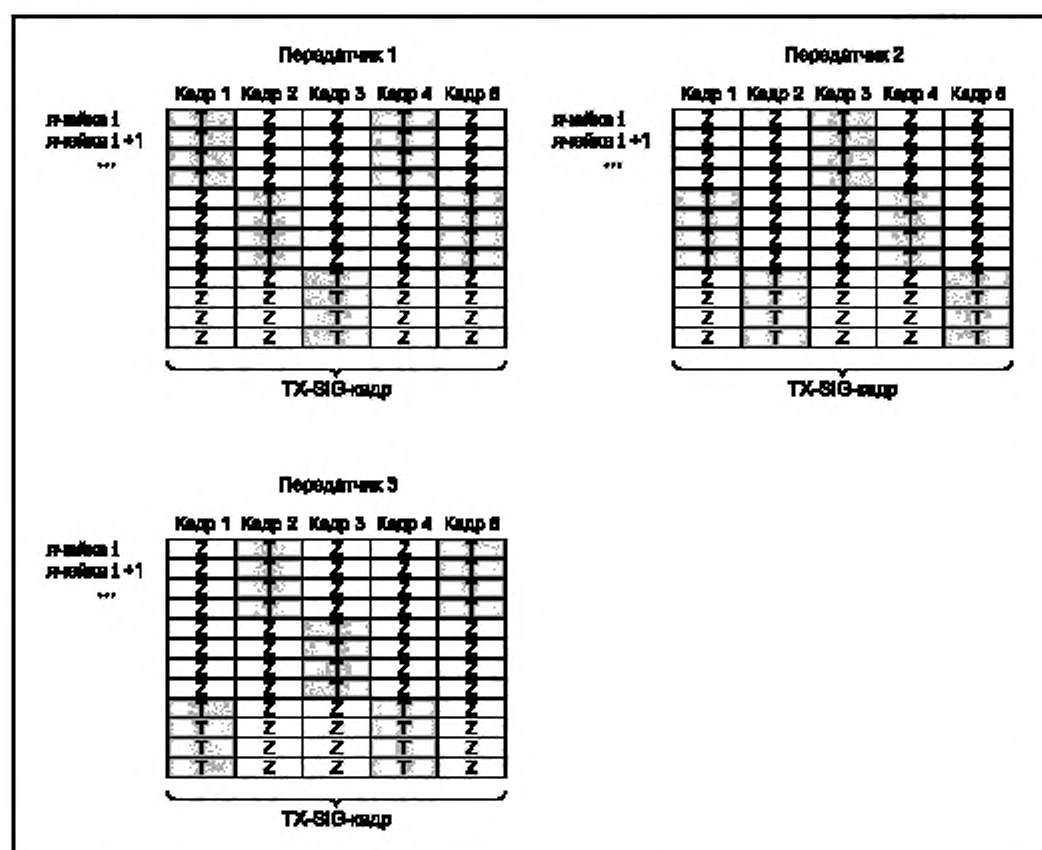
Рисунок 1 — Пример шаблонов дополнительных ячеек, содержащих сигнатуры передатчиков, перед вставкой В-ячеек, для случая M = 3 , N = 4 , L = 5
