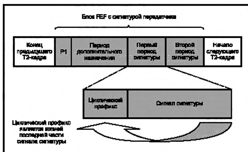
Рисунок 3 — Структура блока FEF с сигнатурой передатчика
