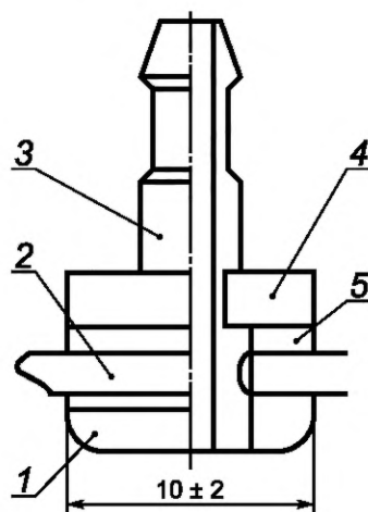
Рисунок 1 — Штуцер
