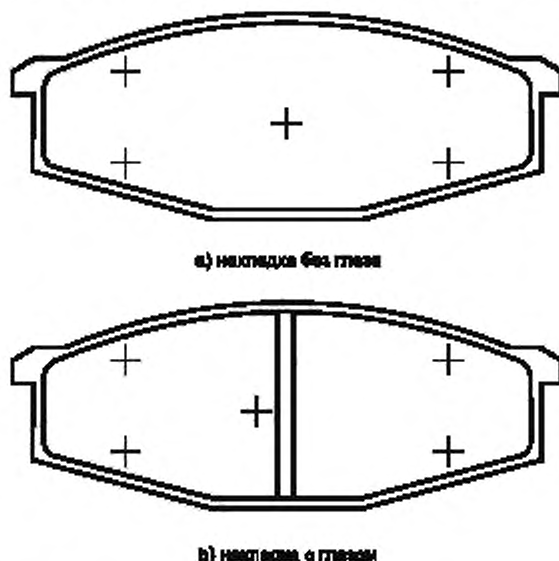
Рисунок 3 — Указания по измерению толщины образца
