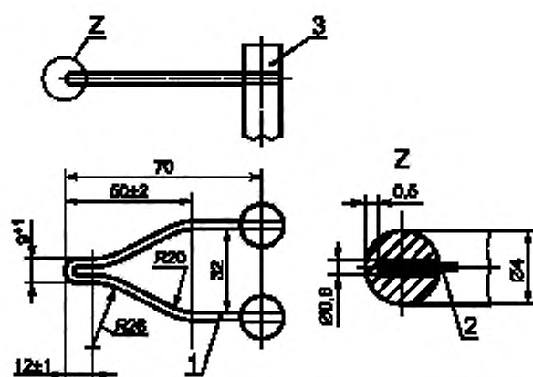
1 — раскаляемая проволока, припаянная к штифту 3; 2 — термонара; 3 — штифт
