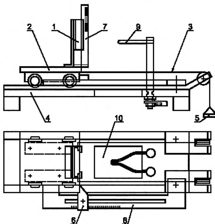
1 — опора для образца; 2 — тележка; 3 — натяжной канат; 4 — груз; 5 — регулируемый упор; 6 — линейка для измерения пламени; 7 — линейка для измерения проникновения; 8 — петля из раскаляемой проволоки (см. рисунок 7); 9 — отверстие в основании
