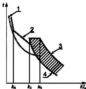
1 — времятоковая характеристика отключения подсоединенного коммутационного аппарата для защиты от сверхтоков; 2 — перегрузочная характеристика; 3 — характеристика отключения; 4 — преддуговая характеристика
