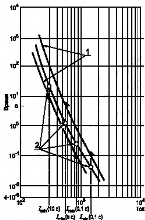
1 — границы зоны времятоковой характеристики; 2 — фактические результаты испытаний
