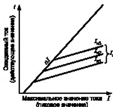
I_{k1}, I_{k2}, I_{k3} — номинальные токи плавких вставок; I_c — максимальное значение пропускаемого тока; n — коэффициент, зависящий от значения коэффициента мощности; nI — асимметричное короткое замыкание
