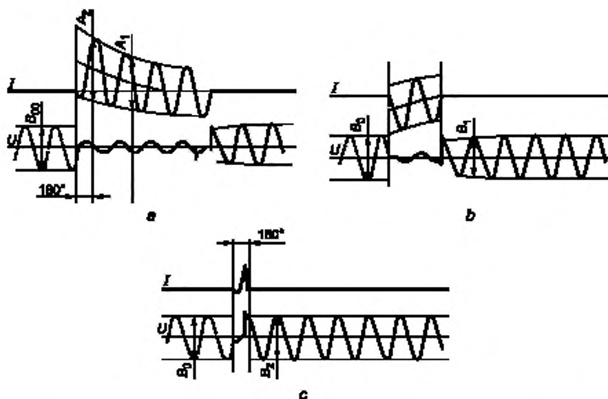
a — осциллограмма при калибровке цепи; b — осциллограмма отключения при образовании дуги после 180^\circ с момента включения; c — осциллограмма отключения при образовании дуги до 180^\circ с момента включения; B_{00} — напряжение калибровки; B_0 — испытательное напряжение;
