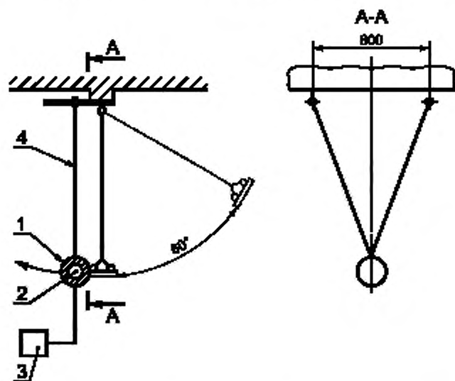
1 — испытательная масса; 2 — акселерометр; 3 — измерительное устройство; 4 — цепи для подвески испытательной массы
