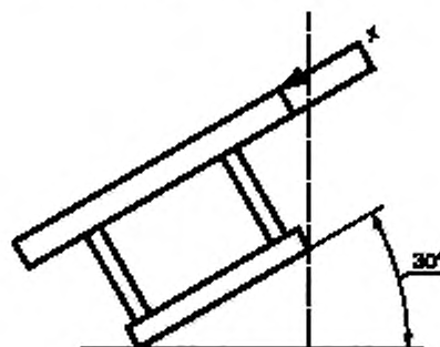
x — задняя кромка верхней части колыбели
