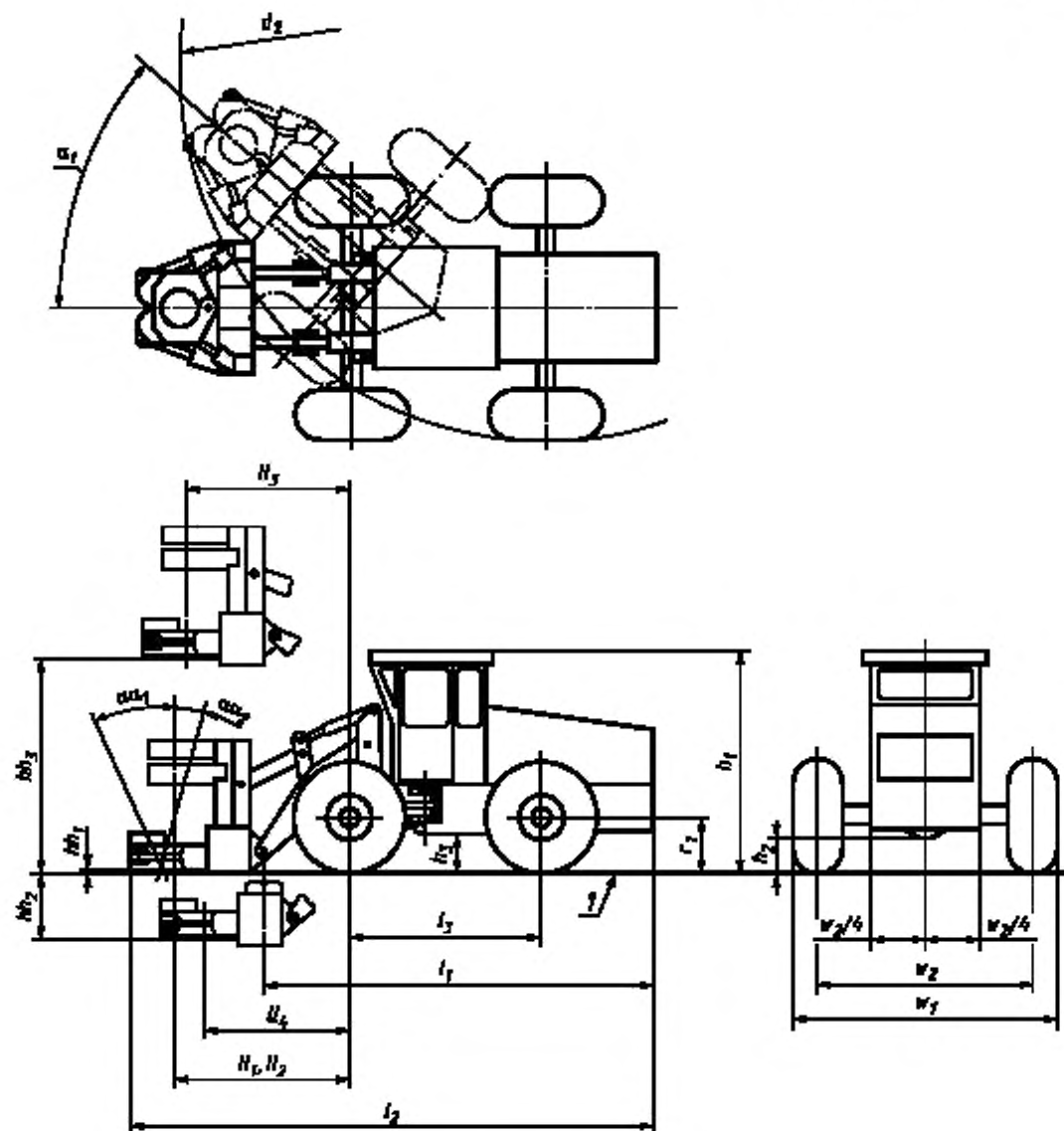
Рисунок 2 — Валочно-пакетирующая машина с фронтальной навеской рабочего органа, колесный тип
