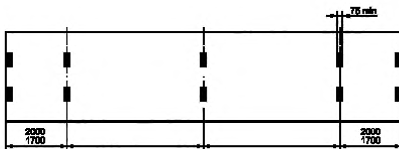
Рисунок Б.3 — Минимальное количество пар опорных (контактных) площадок контейнеров типов IAAA, IAA, IA и IAX без туннеля для захвата типа «шея гуся»
