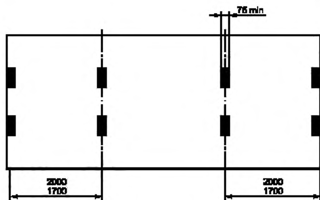
Рисунок Б.2 — Минимальное количество пар опорных (контактных) площадок контейнеров типов ICCC, IC и ICX (при наличии) и контейнеров типов IBVV, IBV, IB и IBX
