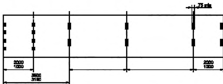
Рисунок Б.4 — Минимальное количество пар опорных (контактных) площадок контейнеров типов IAAA, IAA, IA и IAX с туннелем для захвата типа «шея гуся»
