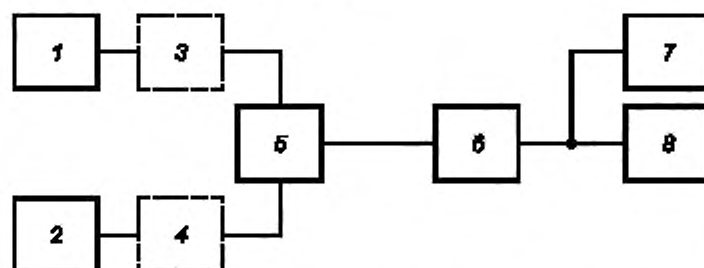
1 2 — генераторы высокочастотных сигналов; 3 4 — фильтр или аттенуатор (при необходимости); 5 — согласующее устройство (эквивалент антенны); 6 — приемник; 7 — вольтметр переменного тока; 8 — эквивалент нагрузки
