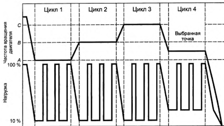
Рисунок Д.1 — Последовательность режимов в испытании ELR
