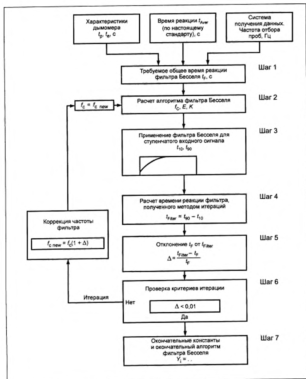
Рисунок К.2 — Пошаговое построение алгоритма фильтра Бесселя
