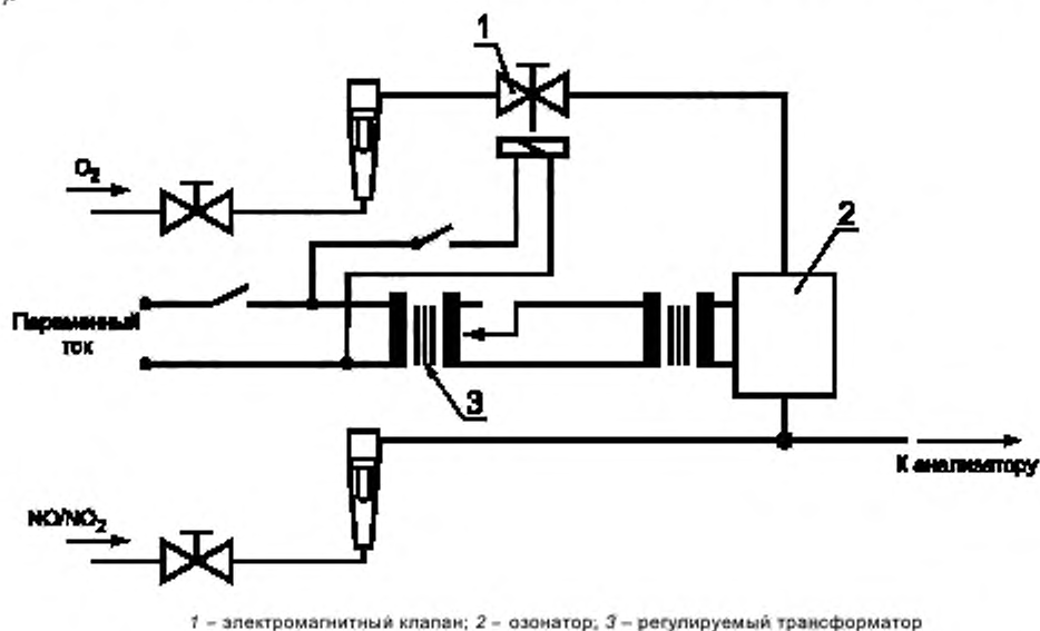
Рисунок Д.4 — Схема устройства для проверки эффективности конвертора \text{NO}_x
