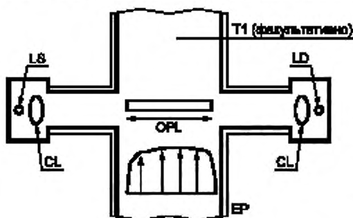
Рисунок Д.21 — Полнопоточный дымометр
