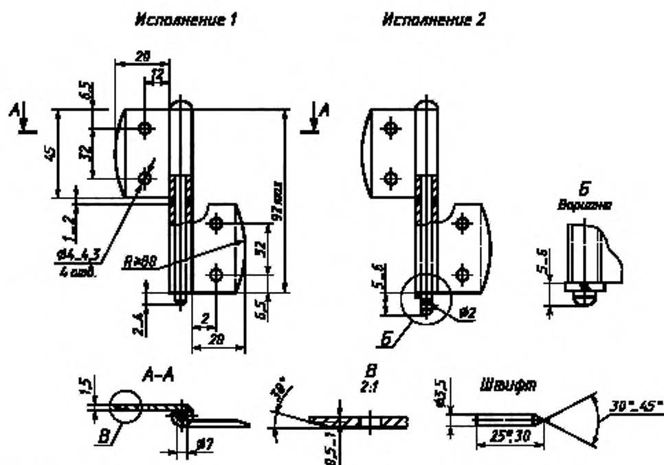
Рисунок Б.17 — Пример врезной петли типа ПВЗ
