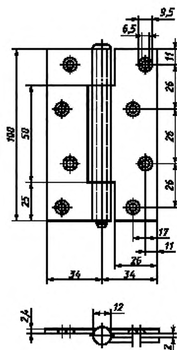
Рисунок Б.19 — Пример резной петли типоразмера ПВ4-100
