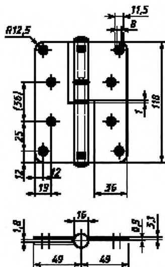
Рисунок Б.2 — Пример накладной петли типоразмера ПН1-110
