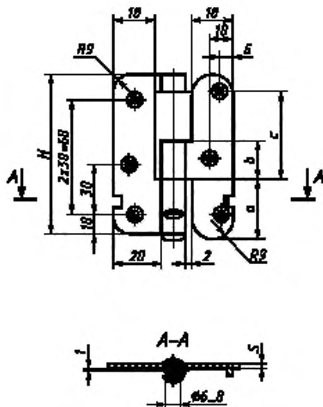
Типоразмер ПН6-80
