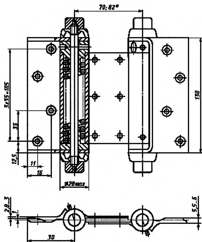
Рисунок Б.14 — Пример накладной петли типа ПН9
