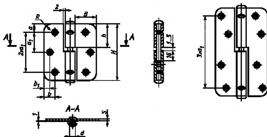
Типоразмер ПНЗ-85
