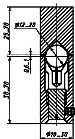
Петля безосевая шаровая верхняя
