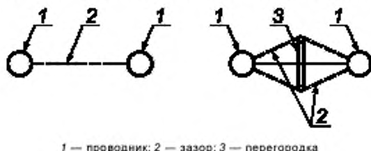
Рисунок С.1 — Измерение зазора
