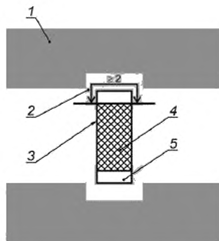
1 — дорожка печатной платы; 2 — паяное соединение между подложкой платы и подложкой компонента ( \geq 2 мм); 3 — компонент с неповреждаемым соединением; 4 — подложка для пайки компонента; 5 — размер подложки для пайки печатной платы установлен по данным изготовителя
