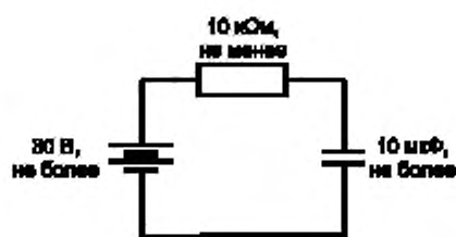
Рисунок А.8 — Простая емкостная цепь
