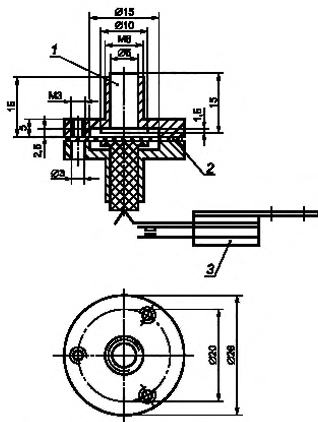
Рисунок В.5 — Пример датчика давления взрыва
