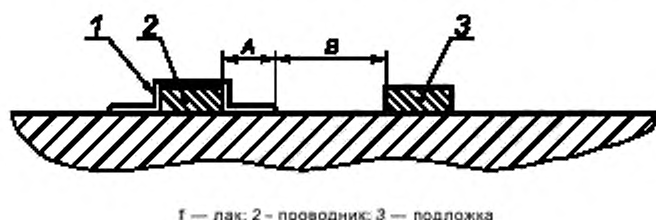
Рисунок С.4 — Измерение сложных расстояний
