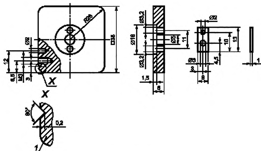
Рисунок В.3 — Держатель проволоки
