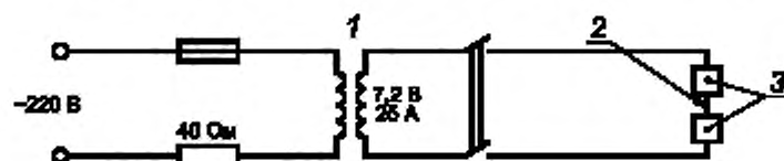
Рисунок В.8 — Принципиальная электрическая схема устройства подготовки вольфрамовых проволочек методом оплавления
