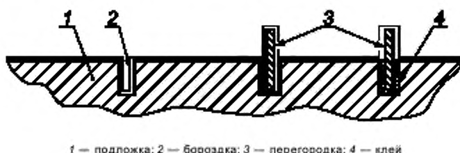
Рисунок С.3 — Измерение длины путей утечки
