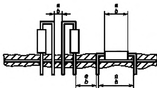
Рисунок б) — Плата с пайкой выступающих выводов резисторов
