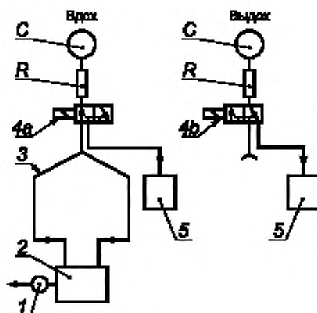
1 — проверяемое устройство для измерения дыхательного объема; 2 — АППАРАТ ИВЛ; 3 — дыхательный контур АППАРАТА ИВЛ; 4a, 4b — пневмораспределитель; 5 — контрольное устройство
