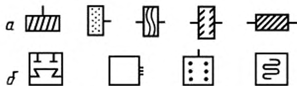
a — фреза, шлифовальный круг, полировальный круг, шевер, фреза цилиндрическая; b — крестовый суппорт, многошпиндельный узел, пульт, магнитная плита
