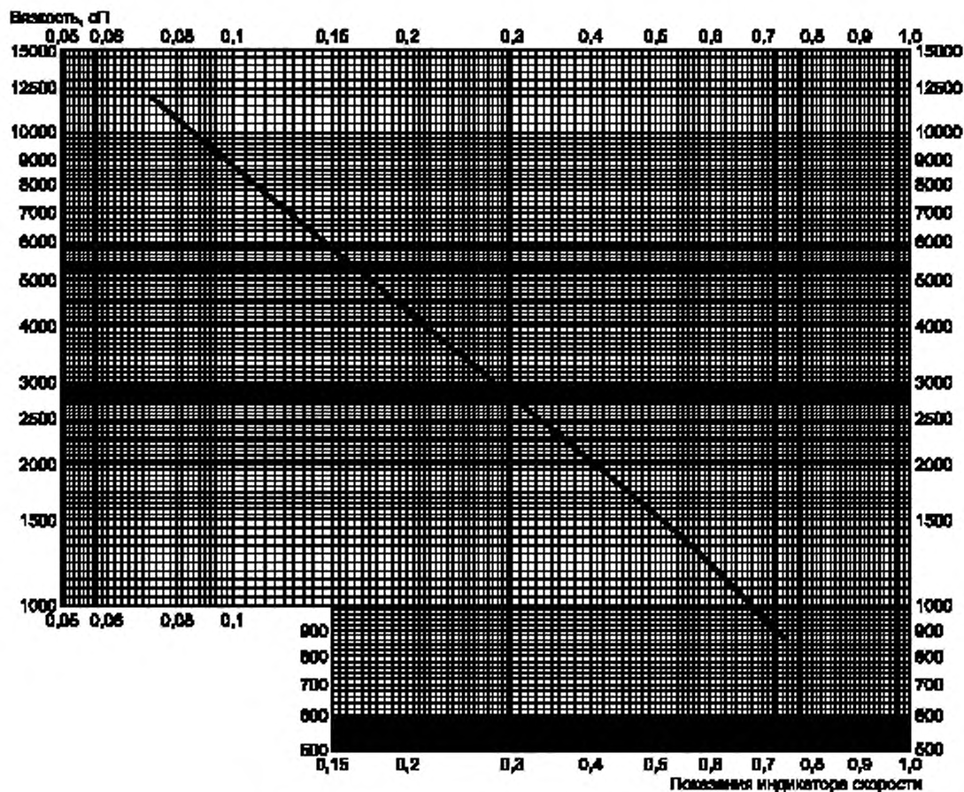
Рисунок Х1.1 — Типичная диаграмма калибровки
