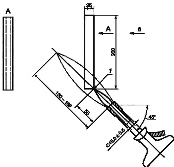
1 — термопара (см. 5.4.6); а — направление воздушного потока, подаваемого после удаления горелки
