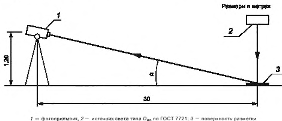
Рисунок 12 Условия определения удельного коэффициента светоотражения при диффузном дневном или искусственном освещении
