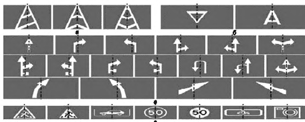
а — для горизонтальной разметки в виде наклонных полос (включая ломаные), ограниченных сплошными одиночными линиями, б — для горизонтальной разметки в виде равнобедренного треугольника, обращенного вершиной к водителю, не окрашенного внутри, и для горизонтальной разметки в виде изображения буквы «А», в — для горизонтальной разметки в виде стрел; г — для горизонтальной разметки в виде изображения дорожного знака
