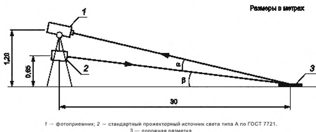
Рисунок 11 — Условия определения удельного коэффициента световозвращения горизонтальной дорожной разметки
