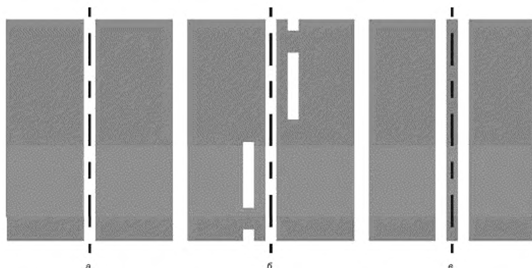
а — для горизонтальной разметки в виде сплошных и прерывистых одиночных линий; б — для горизонтальной разметки в виде сочетания сплошной одиночной линии и прерывистой одиночной линии с соотношением длины штриха к расстоянию между штрихами, равному 3:1; в — для горизонтальной разметки в виде двойной сплошной или прерывистой линии
