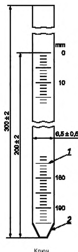
1 — на шкале градуирован каждый миллиметр, числами отмечен внизу каждый сантиметр; 2 — длина сужения от 4 до 8 мм, стенка отверстия минимум 0,5 мм
