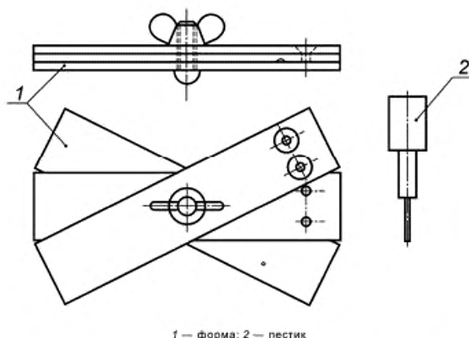
Рисунок 2 — Форма для изготовления образца золы в виде цилиндра
